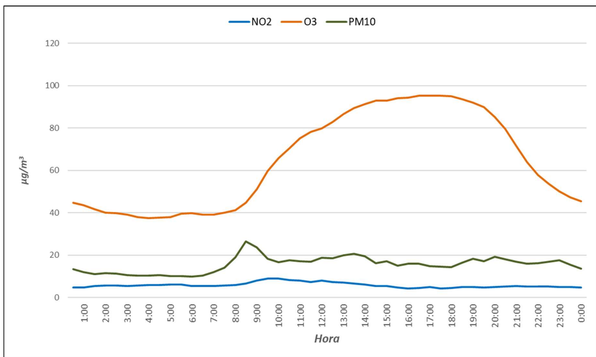
Figura 11. Evolució horària dels contaminants en el dia tipus
