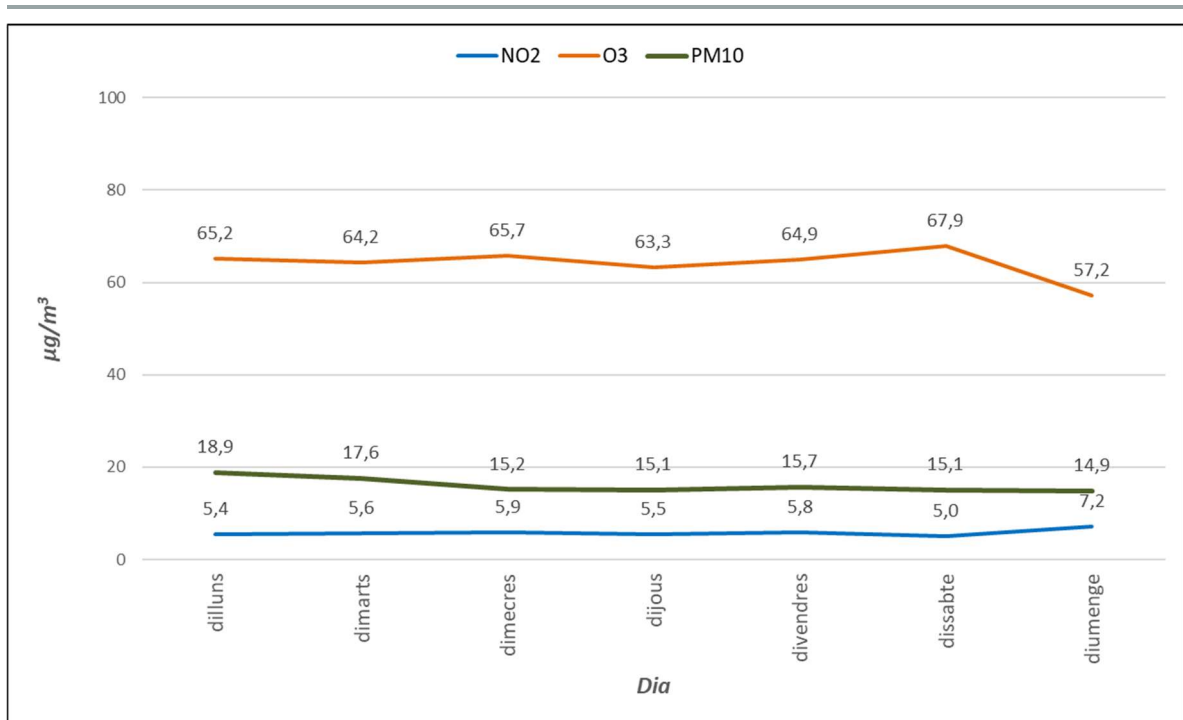
Figura 12. Evolució dels contaminants en la setmana tipus.
