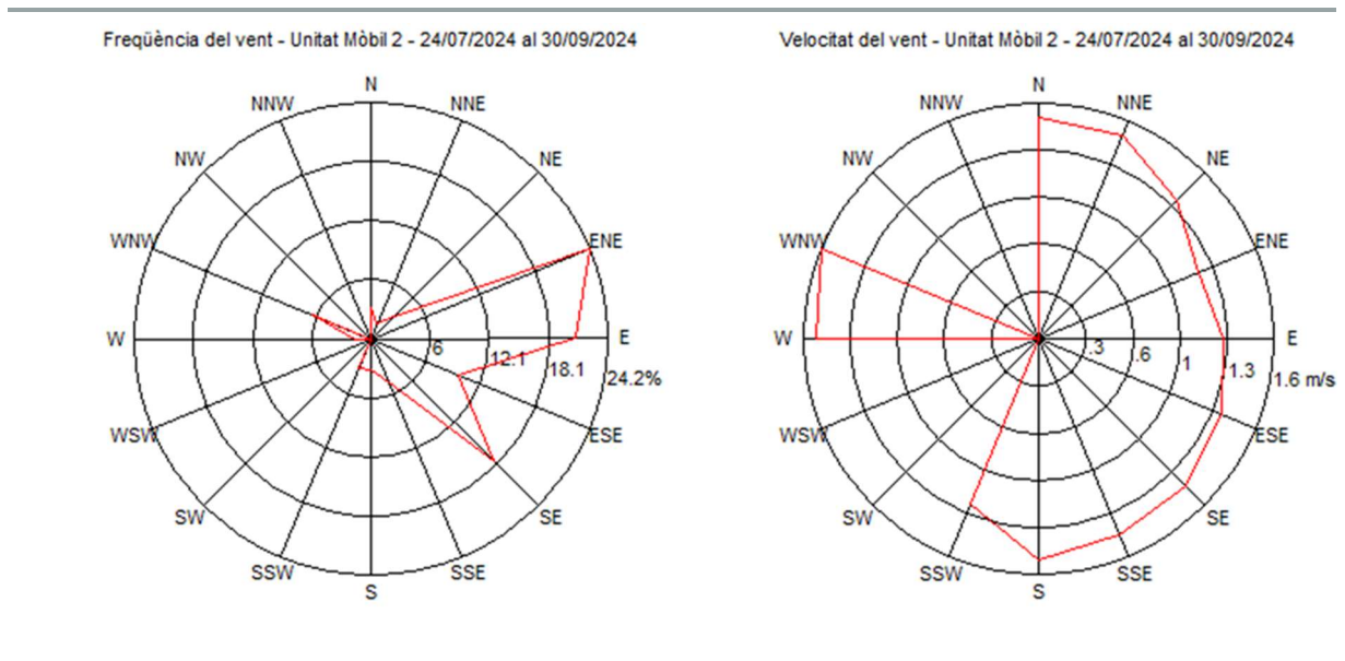
Figura 4. Gràfiques de vent a Sant Climent del Llobregat.
