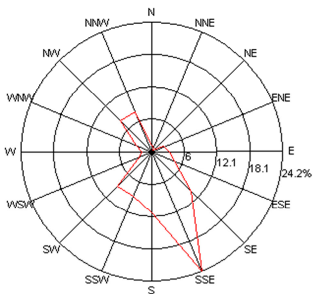
Freqüència del vent - Unitat Mòbil 1 - 01/02/2024 al 08/04/2024
