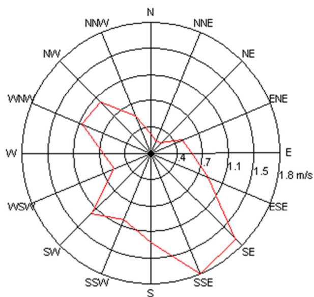
Velocitat del vent - Unitat Mòbil 1 - 01/02/2024 al 08/04/2024
