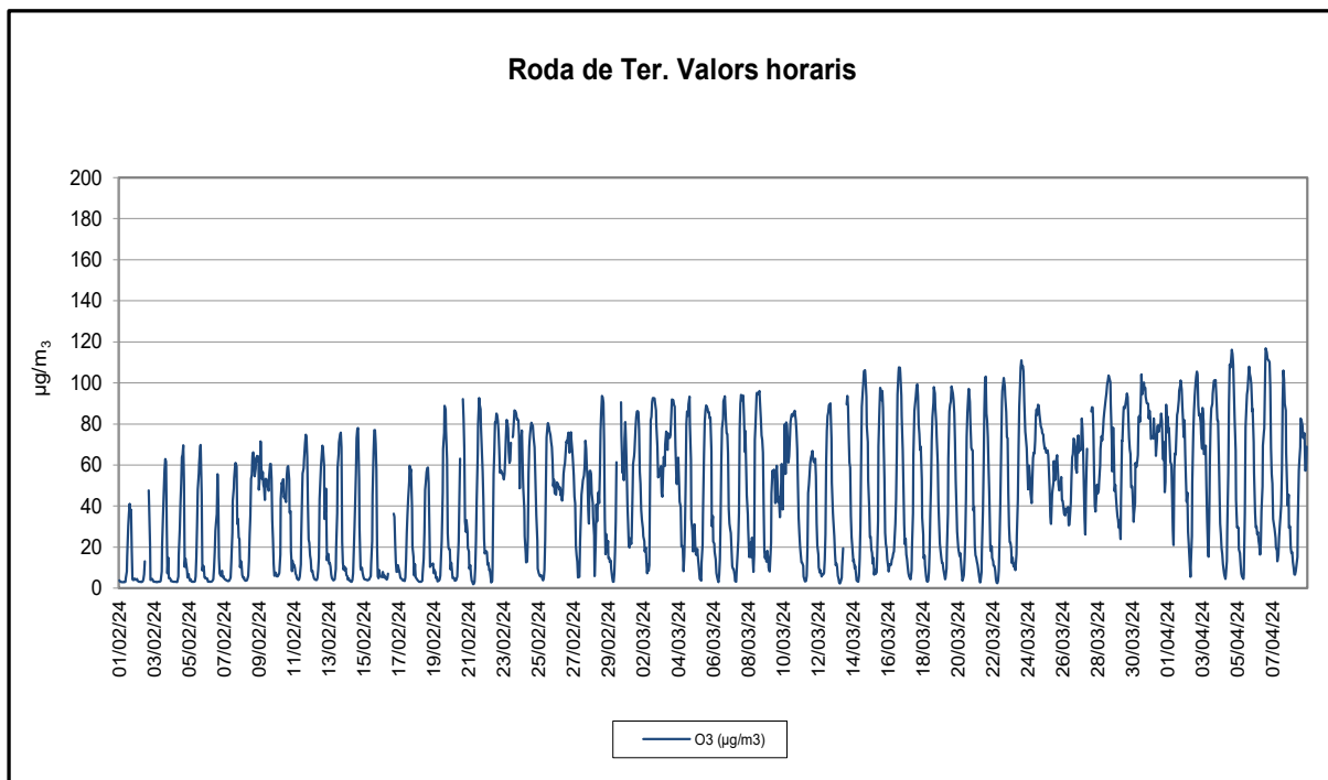
Figura 7. Gràfic dels valors horaris d'ozó
