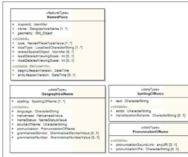
Figura 6. Diagrama de clases UML propuesto en la especificación D2.8.1.3. Fuente: D2.8.1.3 INSPIRE Data Specification on GeographicalNames-Guidelines.
