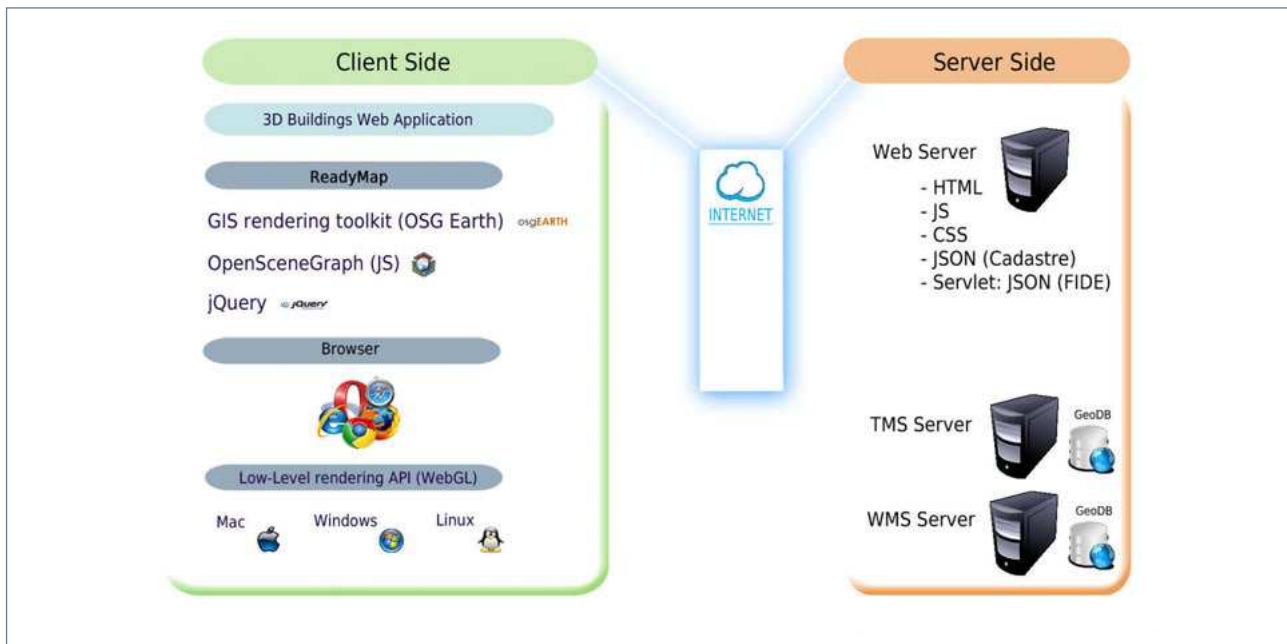
Figura 1. Arquitectura de SOSTRE.
