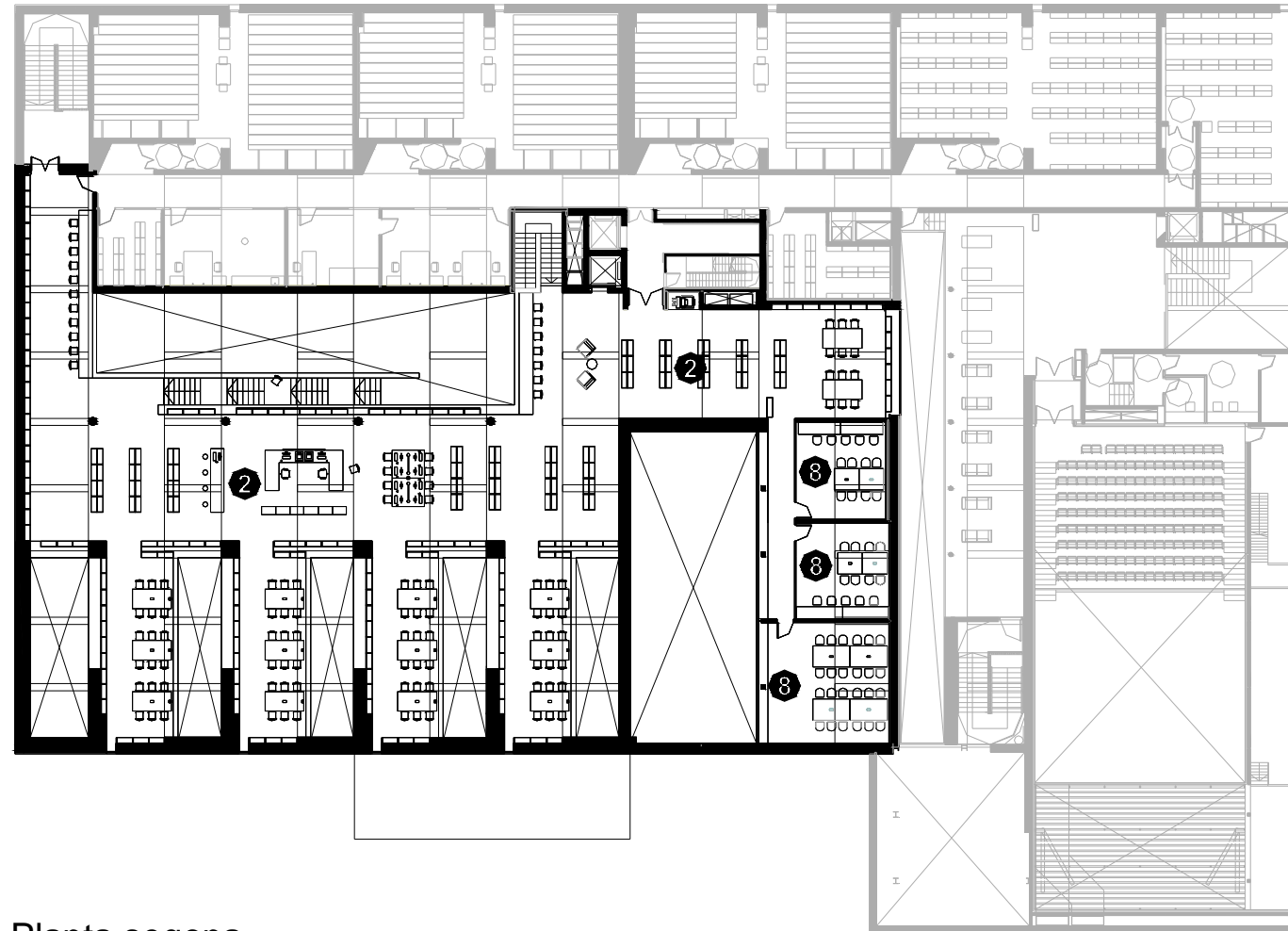
Planta segona
