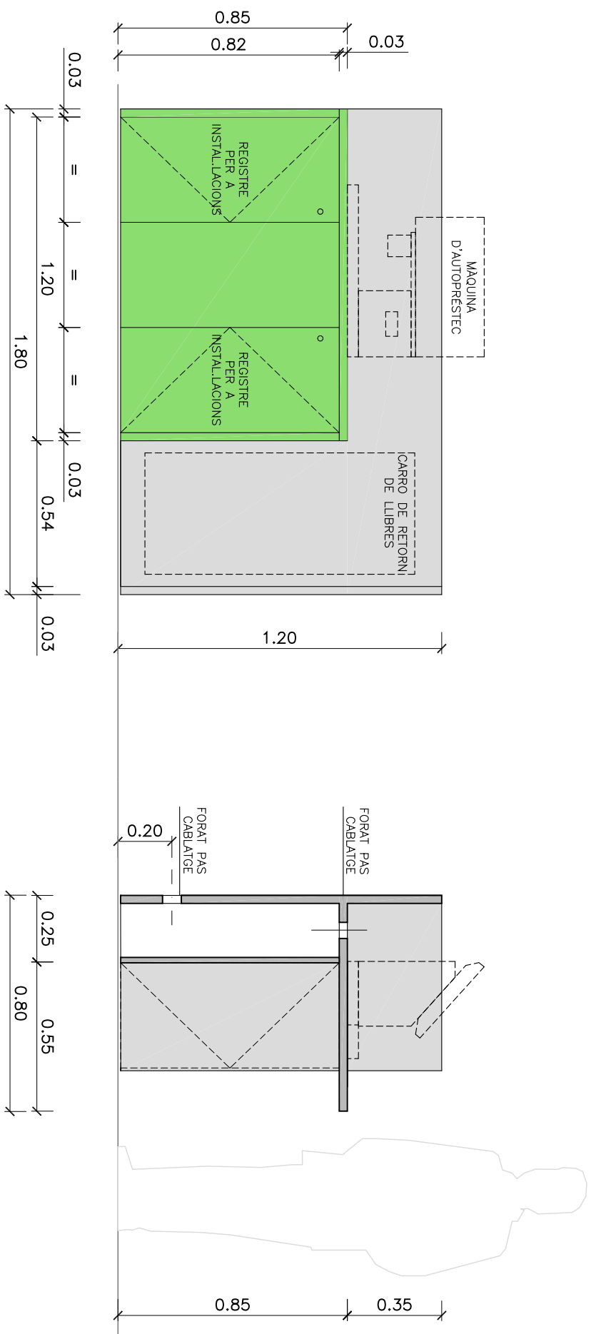
ALÇAT FRONTAL
