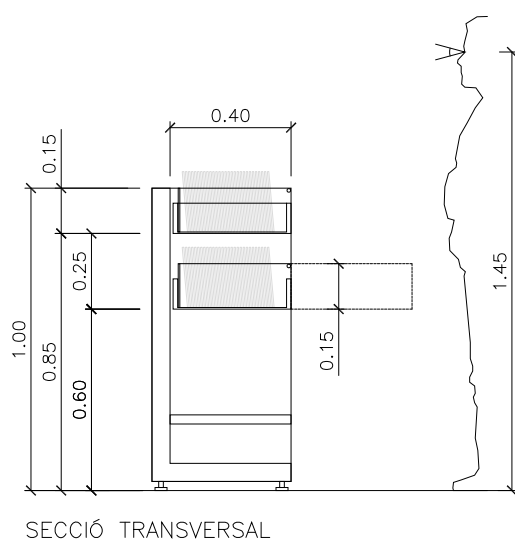
SECCIÓ TRANSVERSAL
