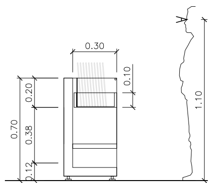
SECCIÓ TRANSVERSAL
