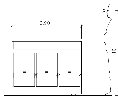
ALÇAT FRONTAL
