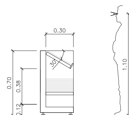
SECCIÓ TRANSVERSAL
