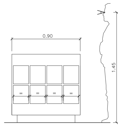
ALÇAT FRONTAL
