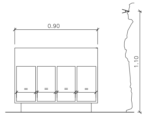
ALÇAT FRONTAL
