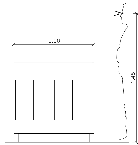
ALÇAT FRONTAL
