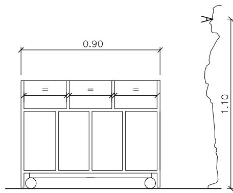
SECCIÓ LONGITUDINAL
