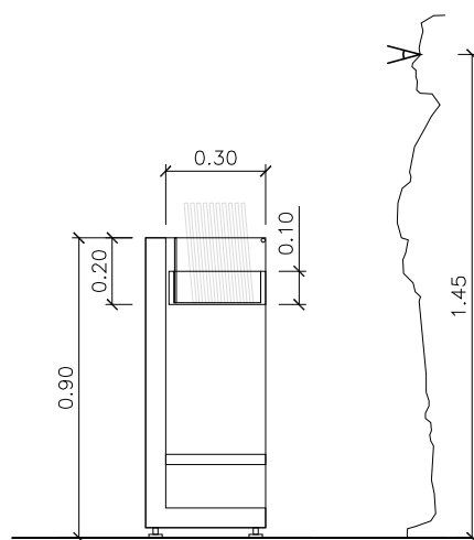
SECCIÓ TRANSVERSAL
