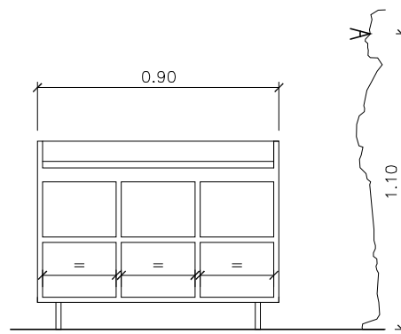
SECCIÓ LONGITUDINAL
