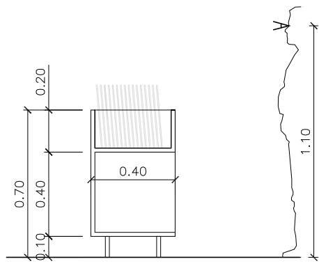
SECCIÓ TRANSVERSAL
