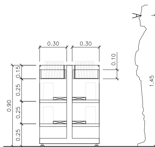
SECCIÓ TRANSVERSAL
