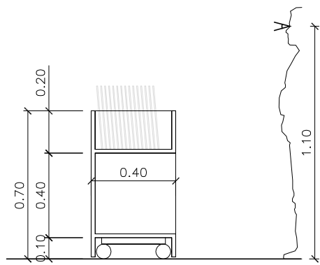
SECCIÓ TRANSVERSAL
