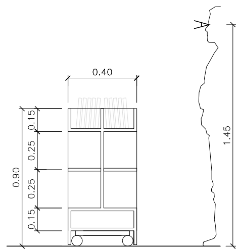
SECCIÓ TRANSVERSAL
