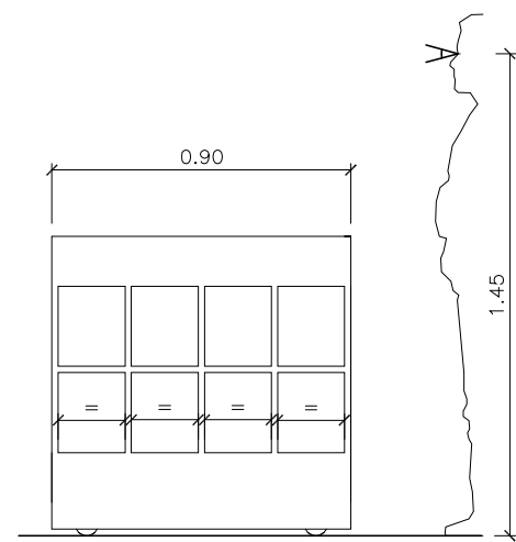
ALÇAT FRONTAL
