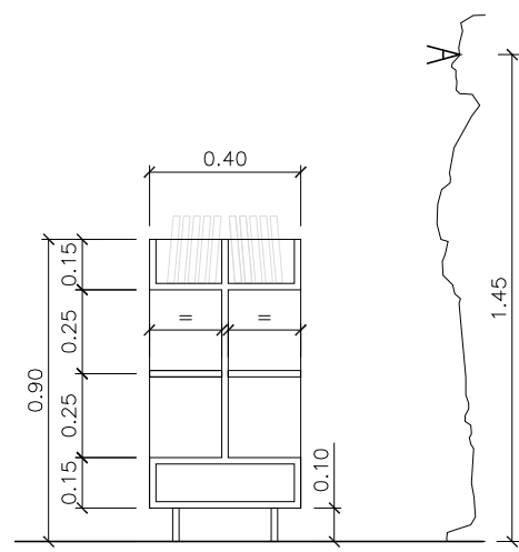
SECCIÓ TRANSVERSAL
