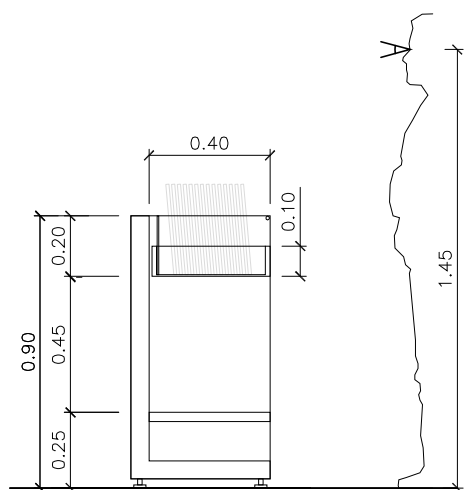
SECCIÓ TRANSVERSAL
