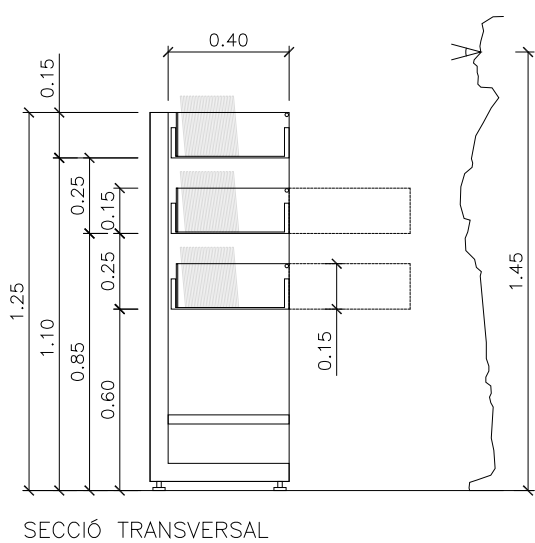
SECCIÓ TRANSVERSAL
